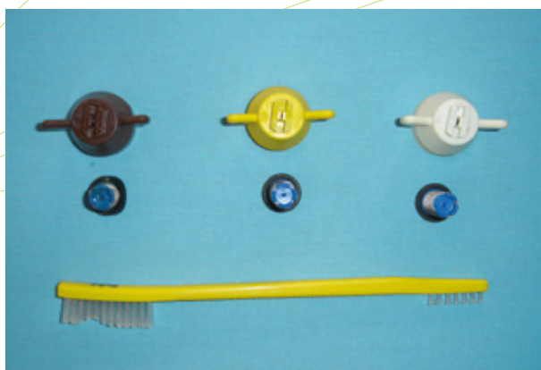
Diverse tipologie di ugello e apposito strumento dedicato alla loro pulizia
